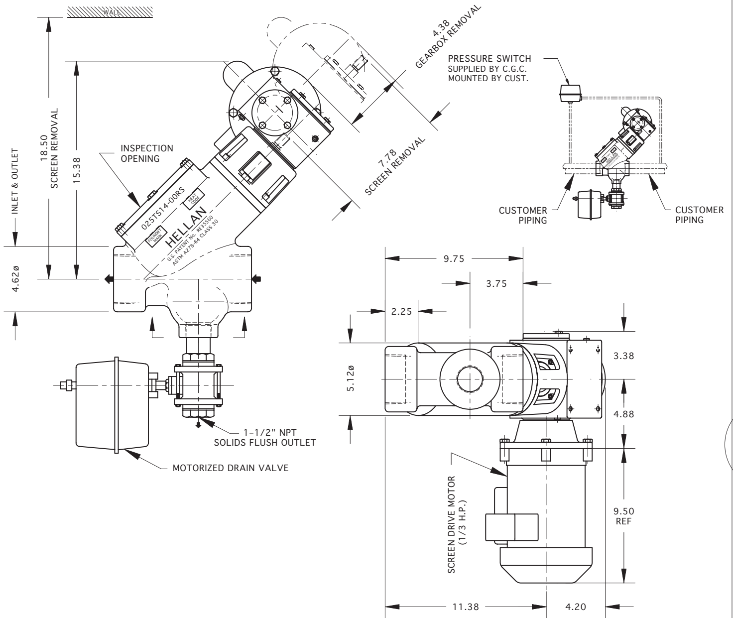
VIEW A-A
