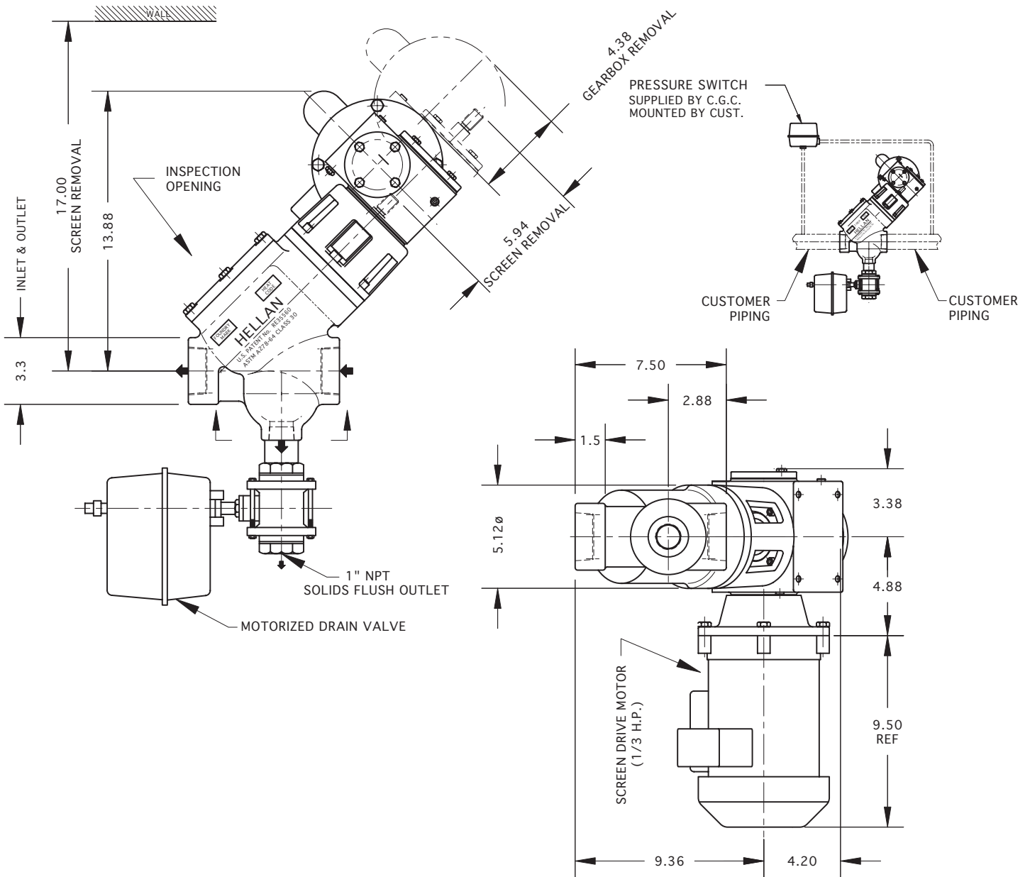
VIEW A-A
